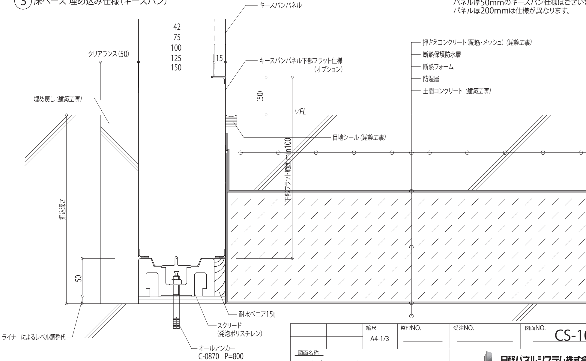
床パネルなし床部詳細図 2 *ご使用になる目的に合わせて仕様を決定してください。
