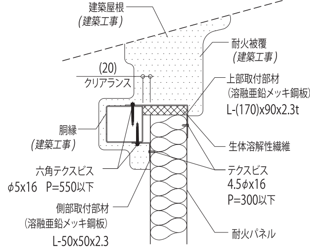
屋根部
