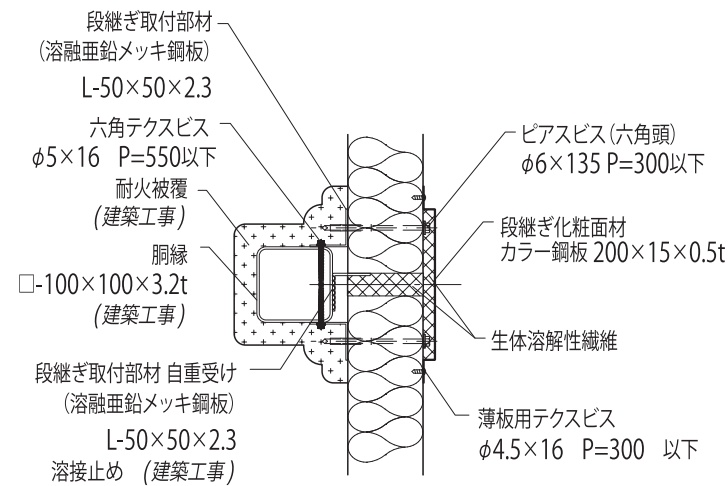
段継ぎ部
