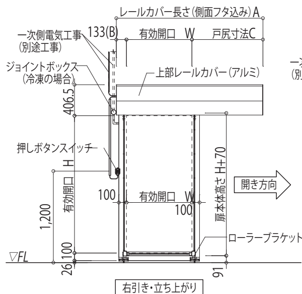
各部寸法
