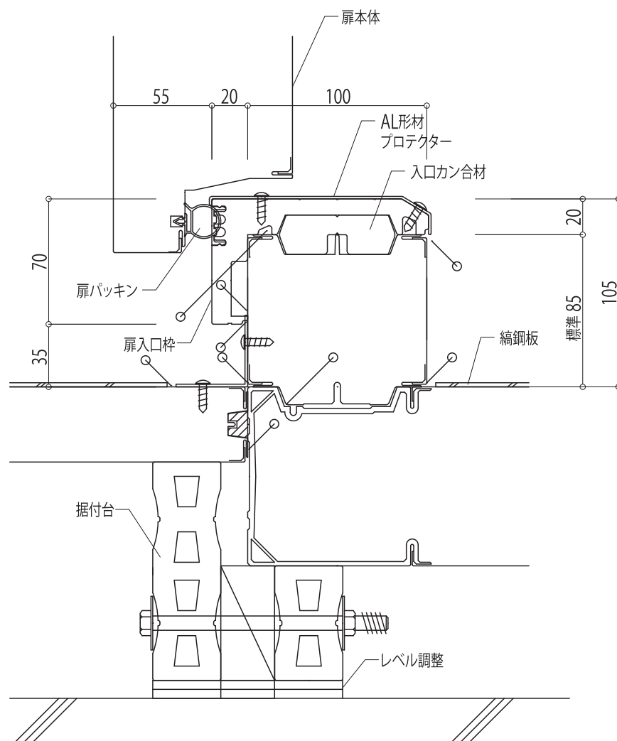
⑦ 床パネル付きドッキングタイプ 間仕切部 立ち上がり四方枠
