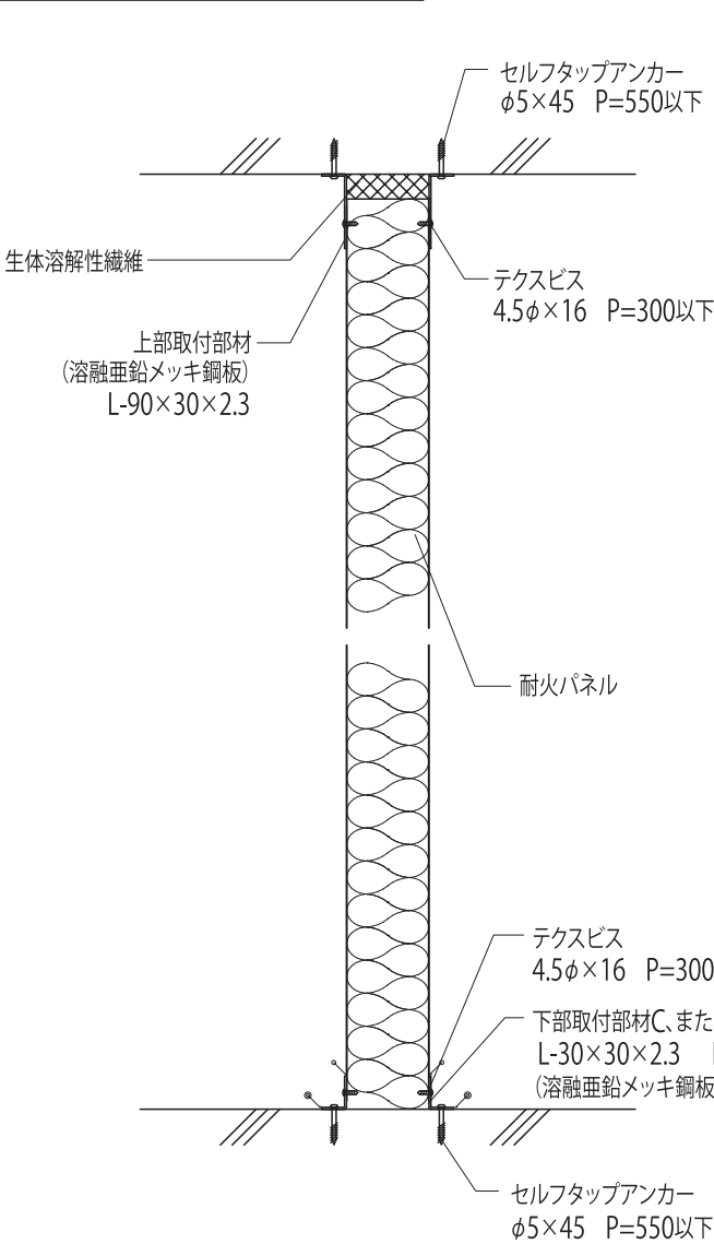
一般断面
